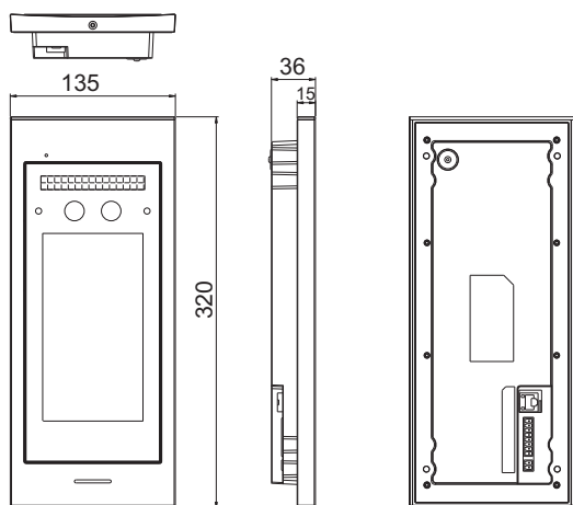
图7 8-T3CS三视图
