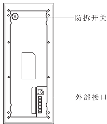
图2 8-T3CS背面视图
