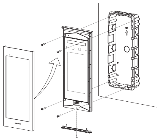
图8 8-T3CS安装图
