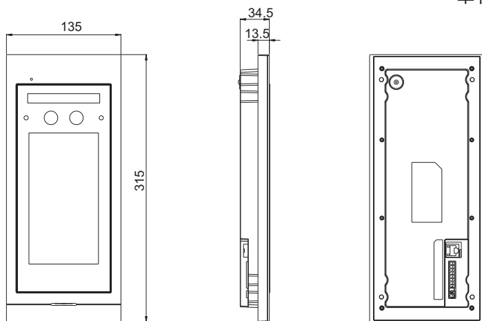
图6 8-K7S三视图
