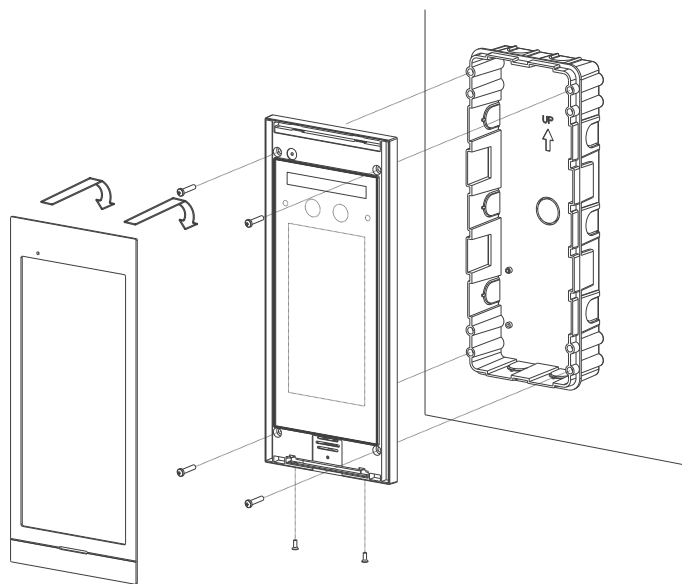
图7 8-K7S安装图
