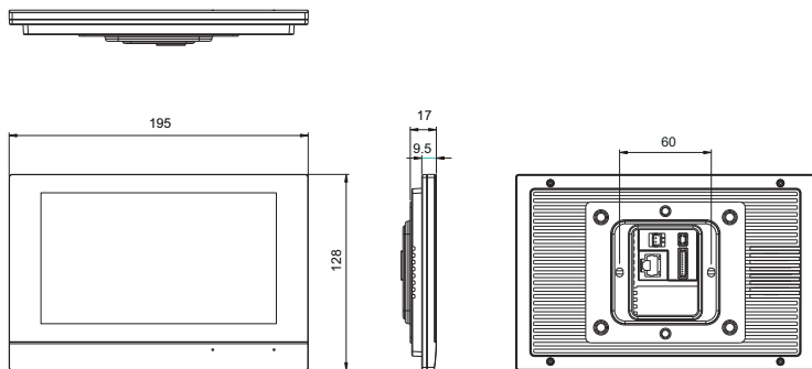
图9 A2MV三视图
