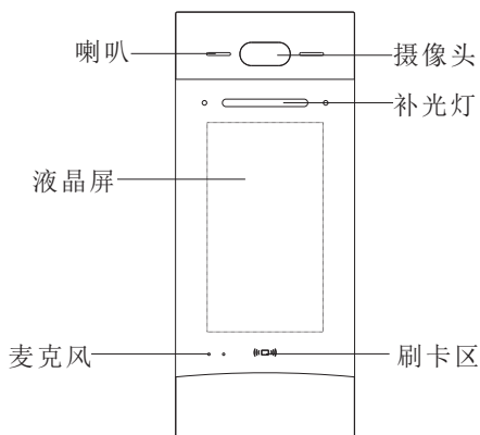
图1 8-K4S正面视图
