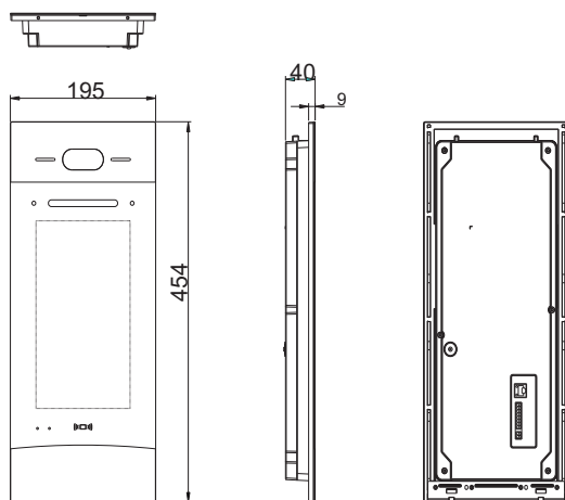
图7 8-K4S三视图
